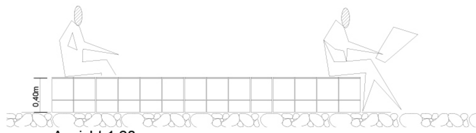
Ansicht 1:20
