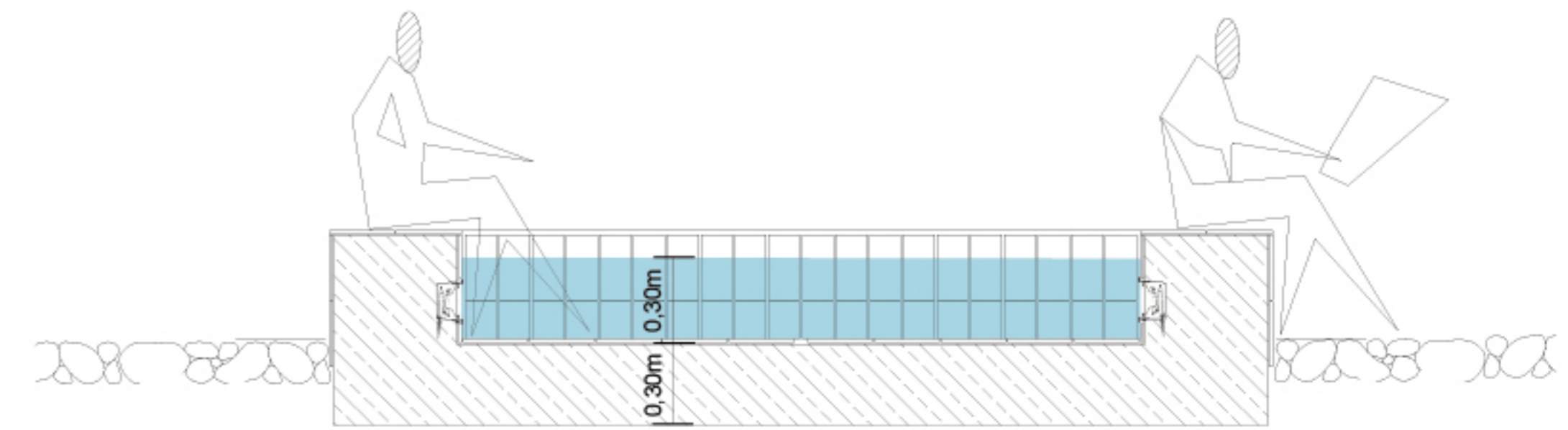
Schnitt 1:20
